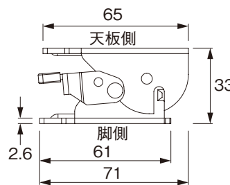
折畳時の寸法図
