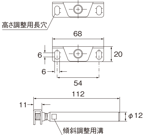
棚加工寸法図
