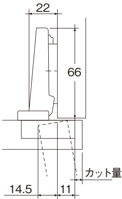
■ F514-1 全かぶせ
