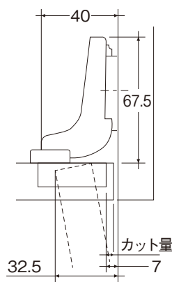
■ F514-3 インセット
