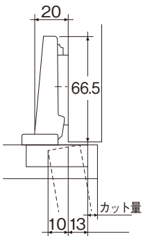
■ F513-1 20mm全かぶせ
