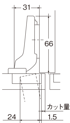
■ F514-2 半かぶせ
