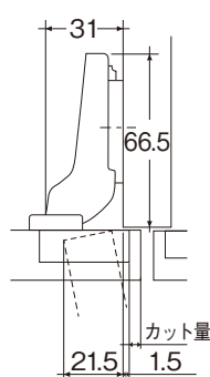
■ F513-3 半かぶせ
