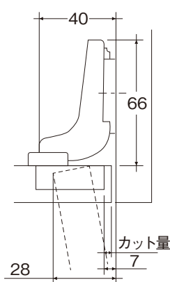
■ F517-3 インセット
