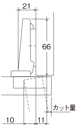
■ F517-1 全かぶせ
