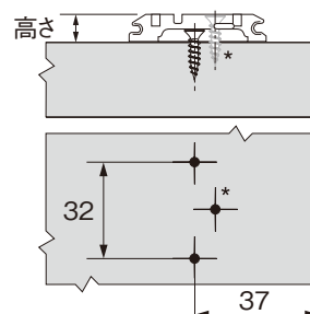
仕様寸法 単位: mm
