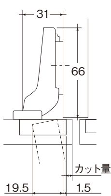
■ F517-2 半かぶせ
