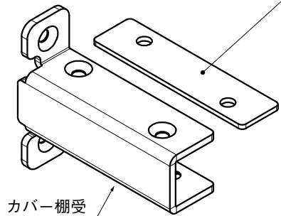
棚板厚 18mm 対応スペーサー（付属品）
