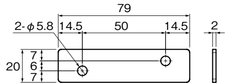
棚板厚18mm対応スペーサー
