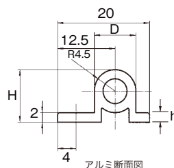
アルミ断面図
